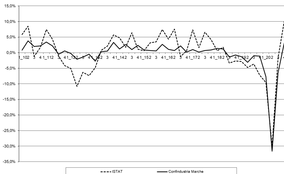
Fig. 6.7 - Indice ISTAT della produzione industriale Italia e indice Confindustria Marche - Gomma e Plastica
